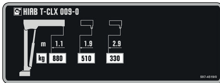
Belastningsskilt HIAB T-CLX 009-0
