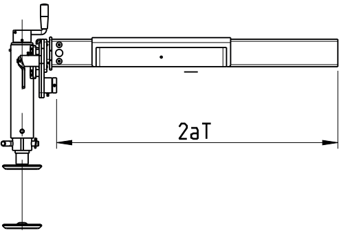
Fundament med opsvingbare støtteben
