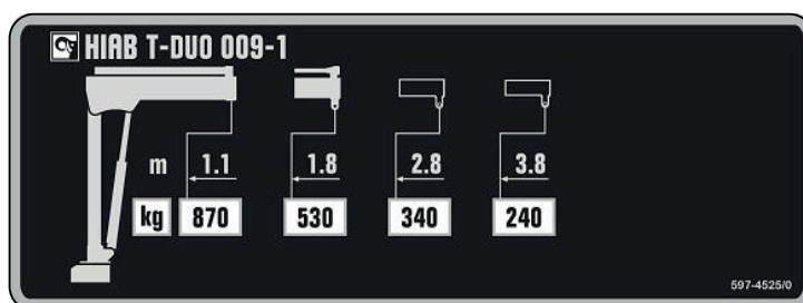
Belastningsskilt HIAB T-CLX 009-1
