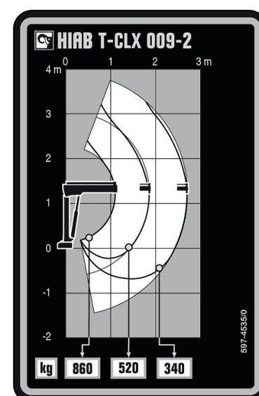
Lastdiagram HIAB T-CLX 009-2
