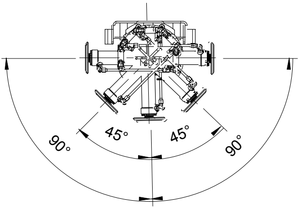
Parkeringsposition for opsvingbar støtteben
