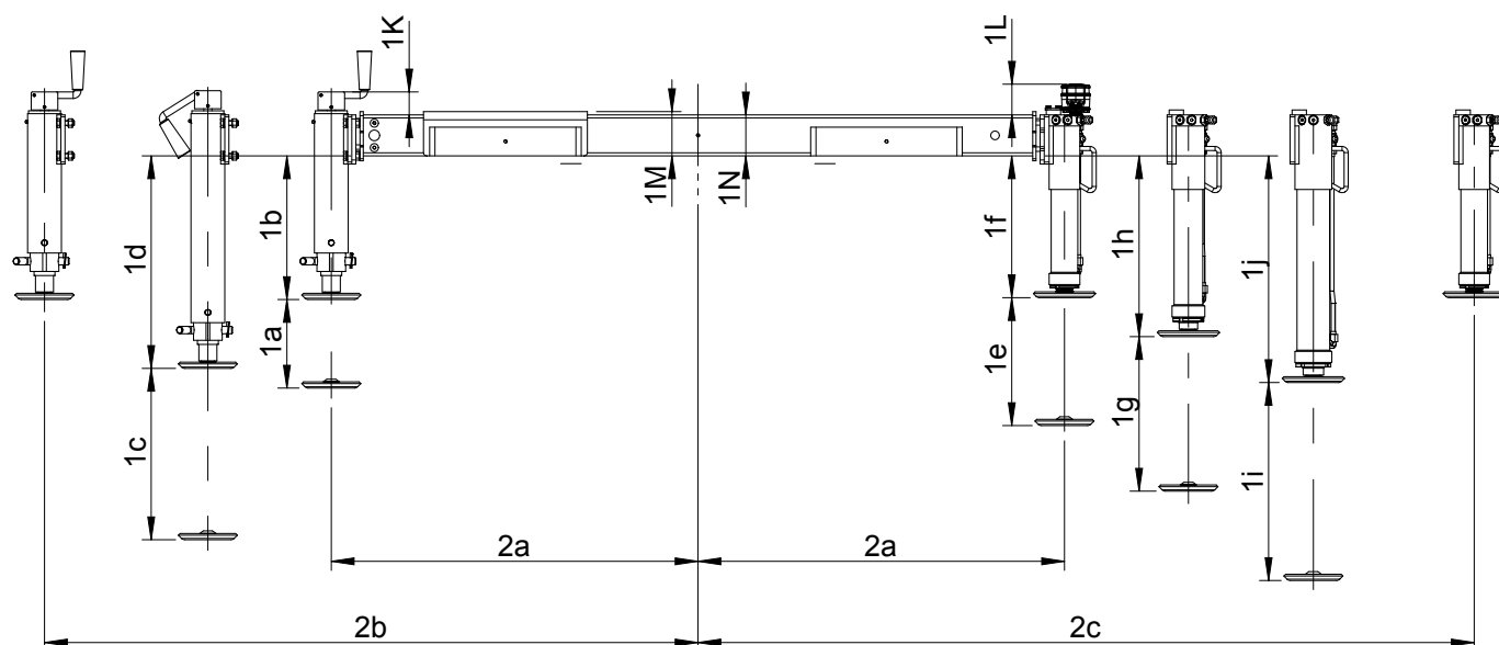
Hydraulisk støtteben
