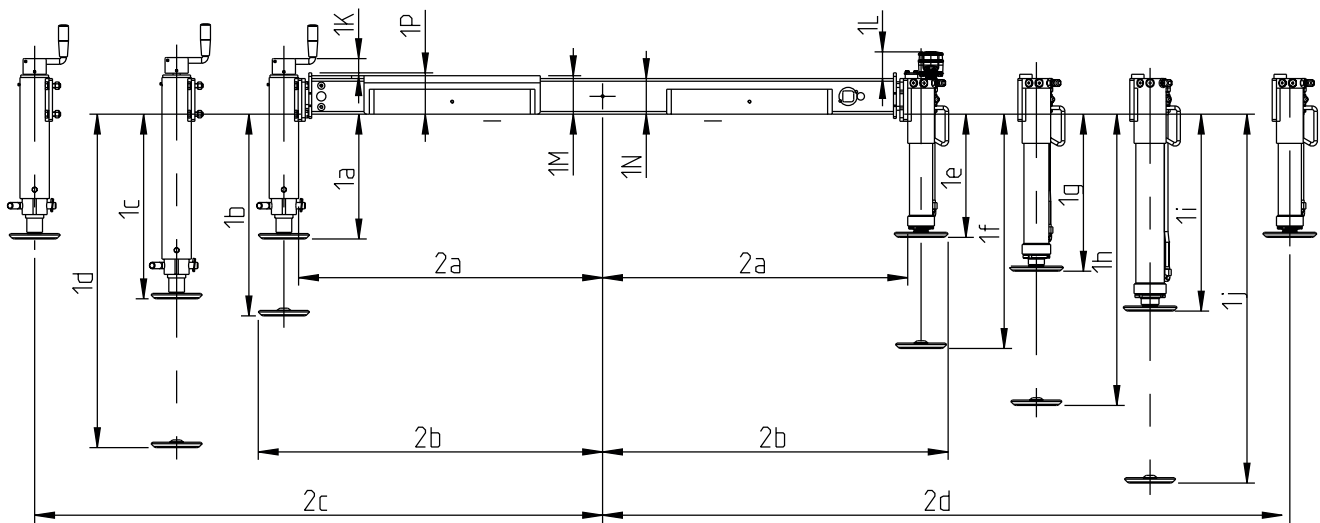
Hydraulisk støtteben
