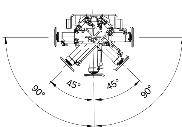
Støtteben med opsving i parkeret position
