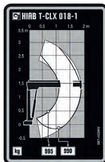
Lastdiagram HIAB T-CLX CE 018-1 CE
