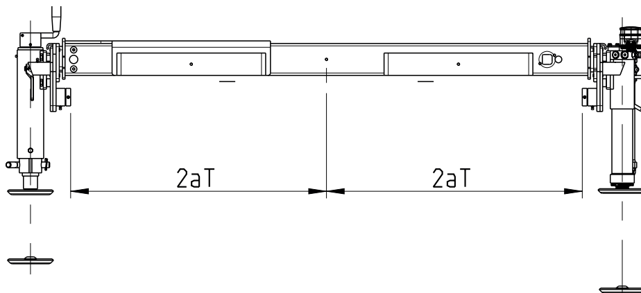
Fundament med opsvingbare støtteben
