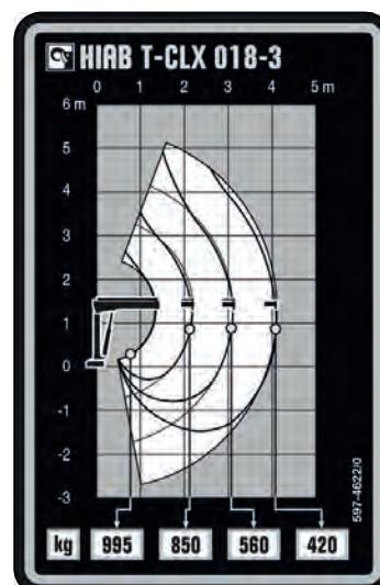
Lastdiagram HIAB T-CLX CE 018-3 CE
