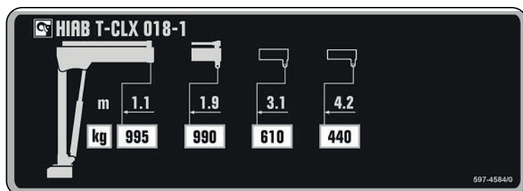
Capacity plate HIAB T-CLX 018-1 CE
