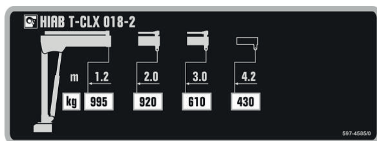
Capacity plate HIAB T-CLX 018-2 CE
