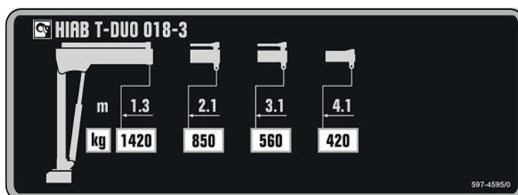
Belastningsskilt HIAB T-DUO 018-3
