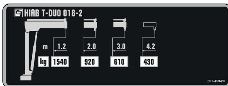
Belastningsskilt HIAB T-DUO 018-2
