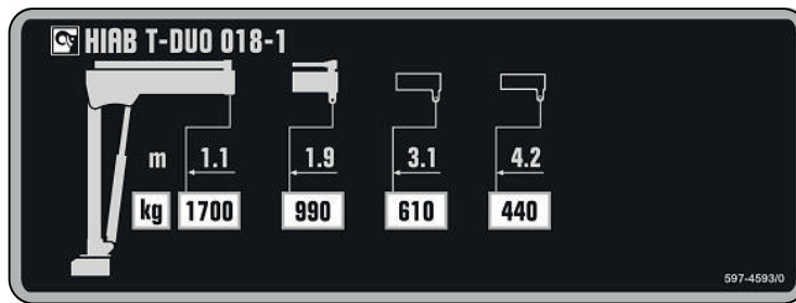
Belastningsskilt HIAB T-DUO 018-1
