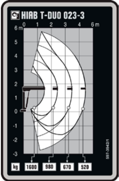
Lastdiagram HIAB T-DUO 023-3
