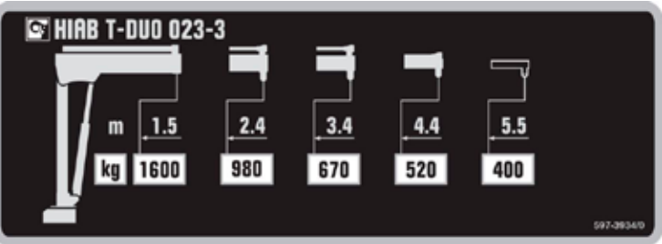
Kapacitetsplade HIAB T-DUO 023-3
