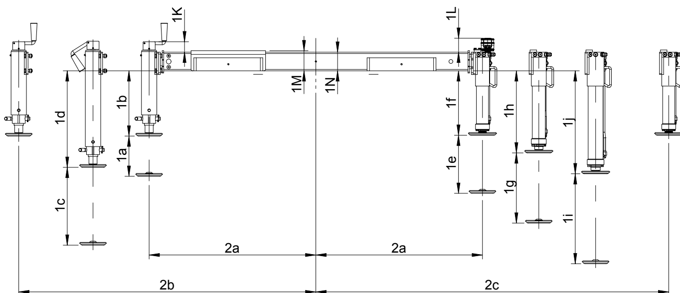
Hydraulisk støtteben
