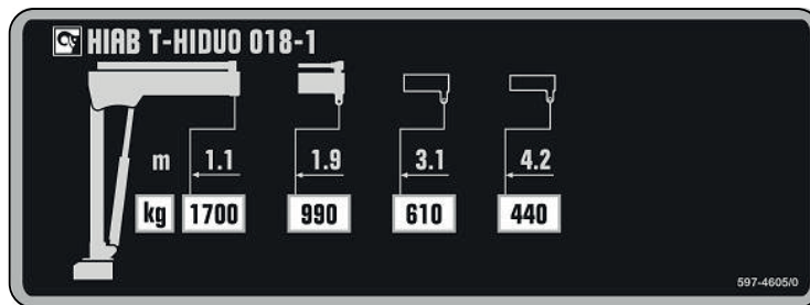
Belastningsskilt HIAB T-HIDUO 018-1
