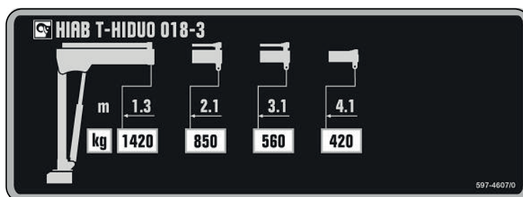
Belastningsskilt HIAB T-HIDUO 018-3
