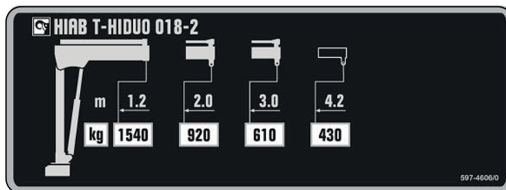
Belastningsskilt HIAB T-HIDUO 018-2
