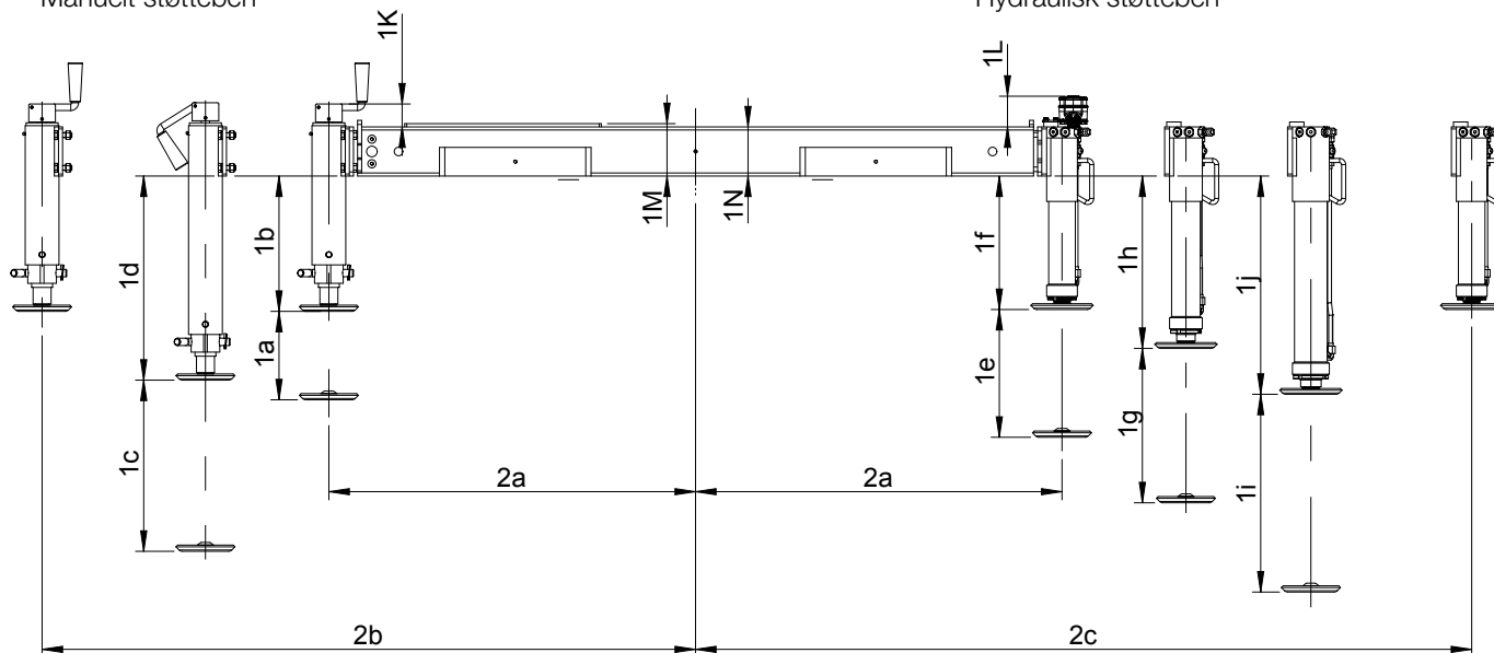
Manuelt støtteben
