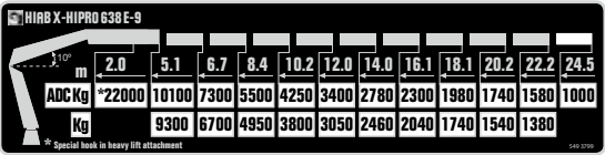
Kapacitetsplade HIAB X-HIPRO 638 E-9
