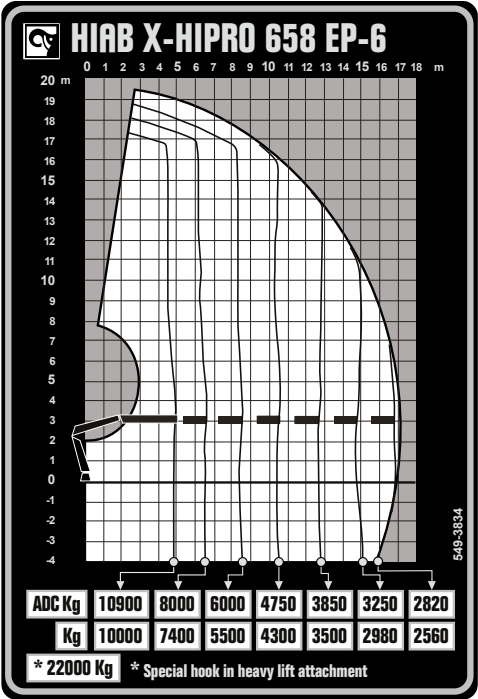
Lastdiagram HIAB X-HIPRO 658 EP-6
